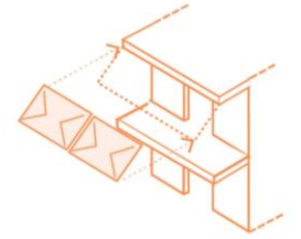
ΕΓΚΑΤΑΣΤΑΣΗ ΚΑΤΑΚΟΡΥΦΟΥ ΣΥΣΤΗΜΑΤΟΣ ΗΛΙΟΠΡΟΣΤΑΣΙΑΣ
